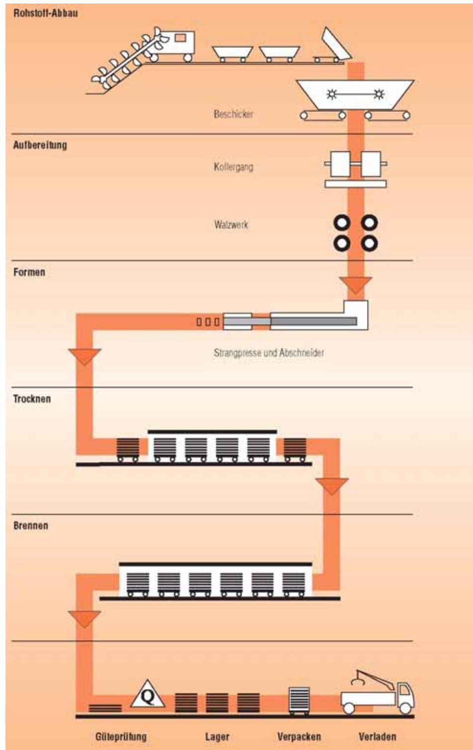
Abbildung 1: Schematische Darstellung der Ziegel-Produktion
